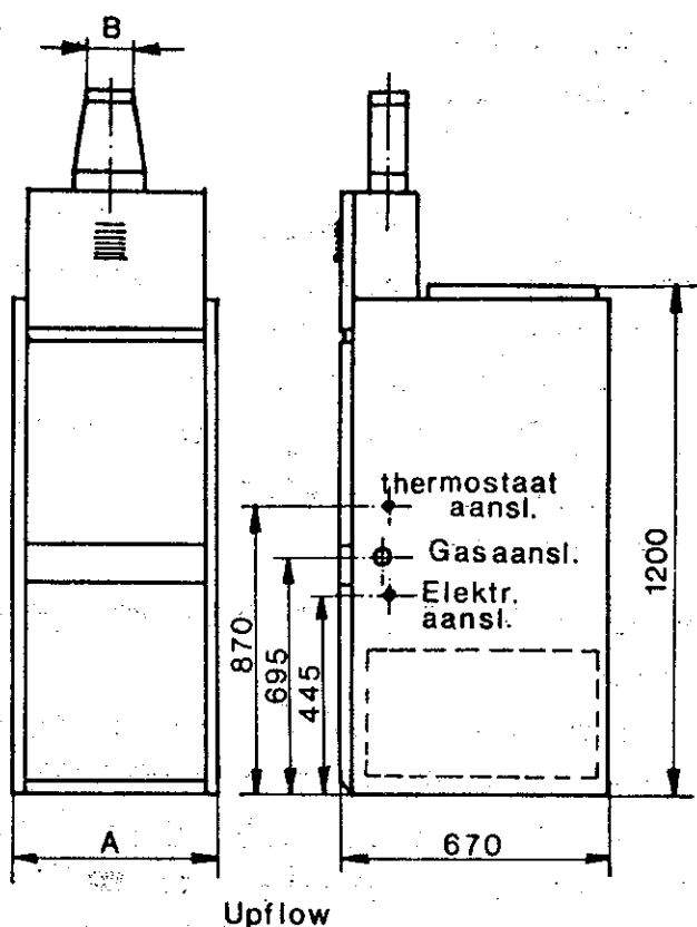
Upflow Figuur 4 Aansluitpunten luchtverhitter.
