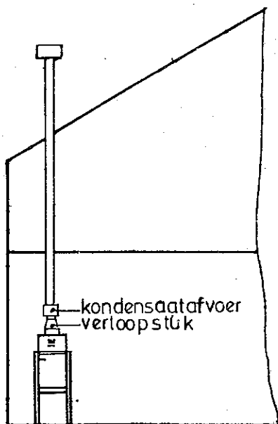
Fig. 3a : inbouw kondensaatafvoer bij een rookgasafvoersysteem zonder bochten in de stookruimte
