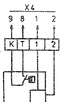
4-draads klokthermostaat zwevend contact
