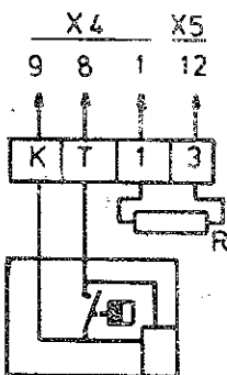
2-draads klokthermostaat Ioff Therm. R(5Watt)
