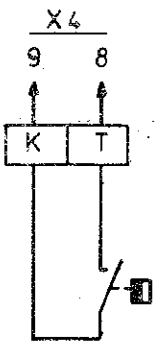
kamerthermostaat (standaard)
