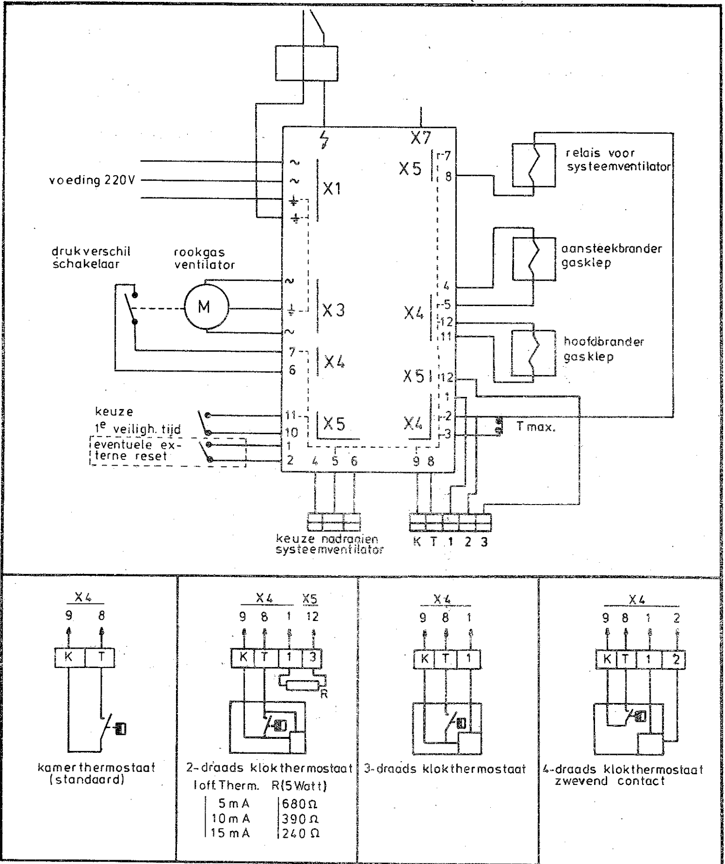
Fig. 9 : Aansluitschema besturingskast Philips MCBA 0211.
