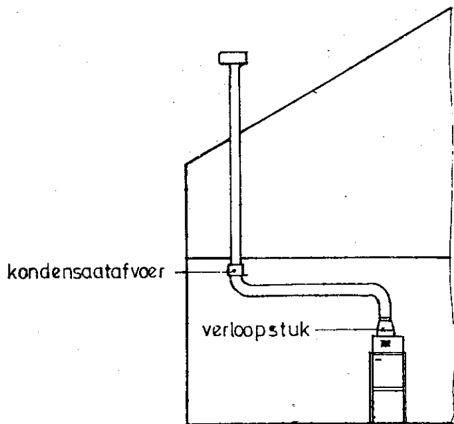
Fig. 3b : inbouw kondensaatafvoer bij een rookgasafvoersysteem met bochten in de stookruimte
